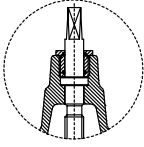
DN40 / DN200 O-Ring Seal O-Ring Sızdırmazlık
